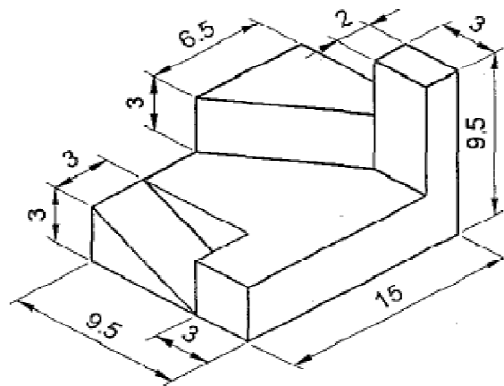
COTAS EM mm ESCALA 5 / 1
