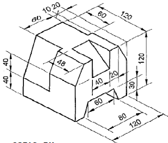
COTAS EM mm ESCALA 1 / 2
