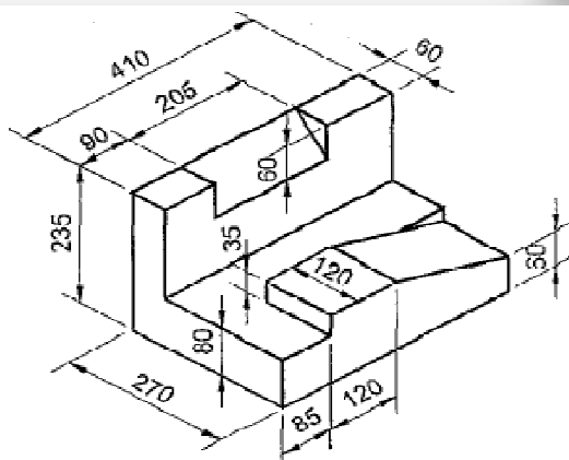
COTAS EM mm ESCALA 1 / 5
